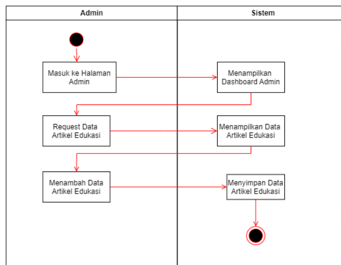
Gambar 3. 7 Admin Tambah Data Edukasi
