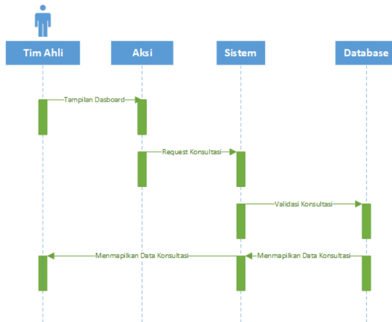
Gambar 3. 31 Sequence Melihat Data Konsultasi
