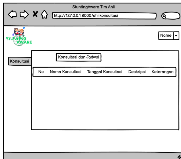
Gambar 3. 41 Ahli Melihat Data Konsultasi
