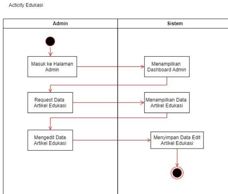
Gambar 3. 8 Admin Edit Edukasi
