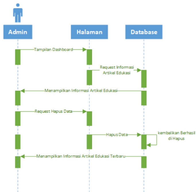
Gambar 3. 21 Admin Hapus Data Edukasi
