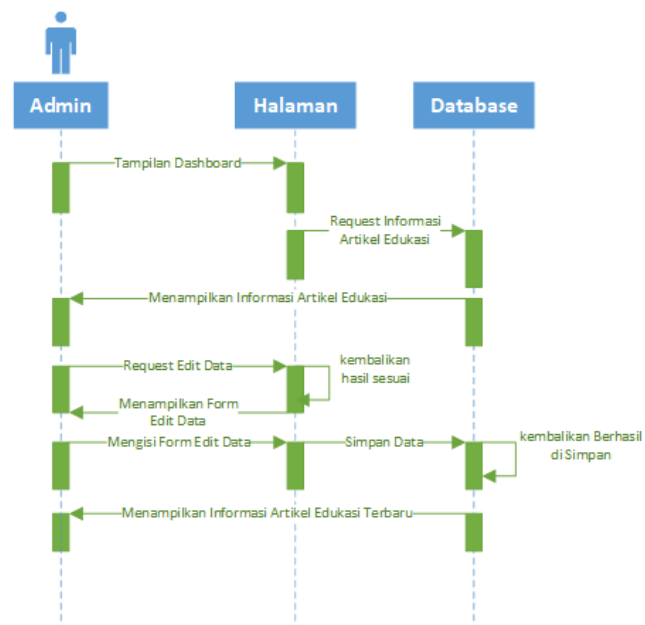
Gambar 3. 20 Admin Edit Edukasi
