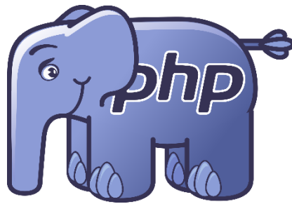
Gambar 2. 6 PHP
