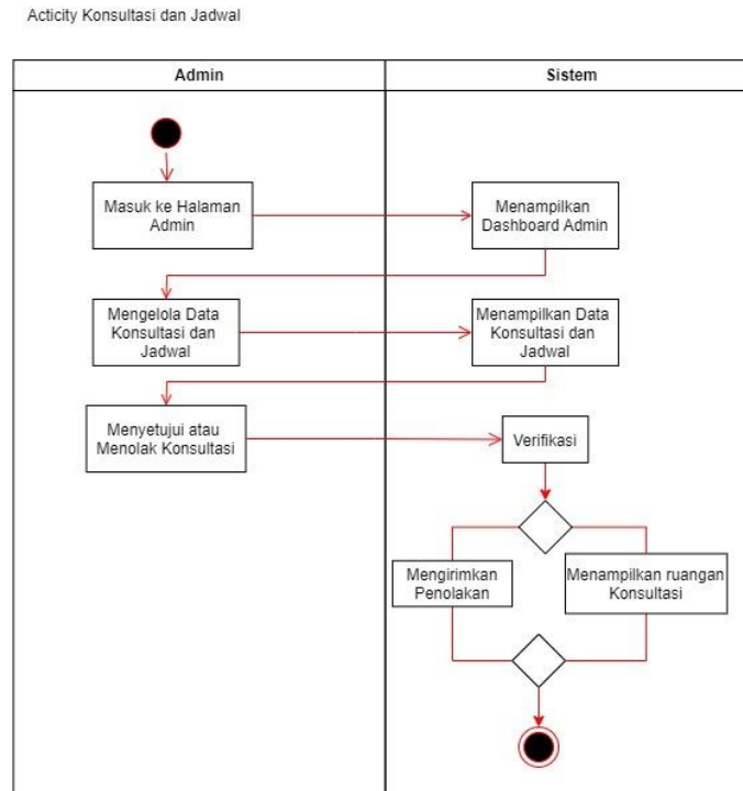
Gambar 3. 10 Activity Admin Konsultasi
