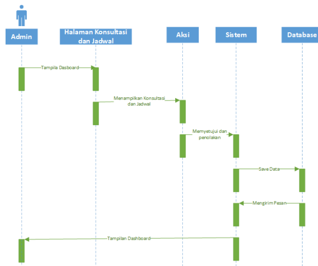
Gambar 3. 22 Sequence Admin Konsultasi
