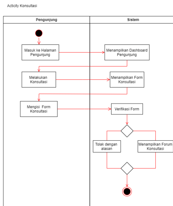
Gambar 3. 14 Activity Konsultasi Pengunjung
